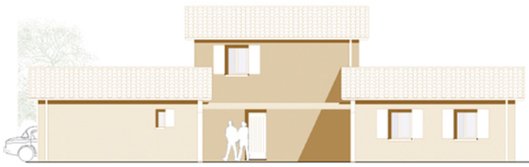
FAÇADE SUD-EST
